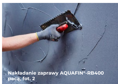
Uszczelnianie elementów budowlanych stykających się z gruntem
